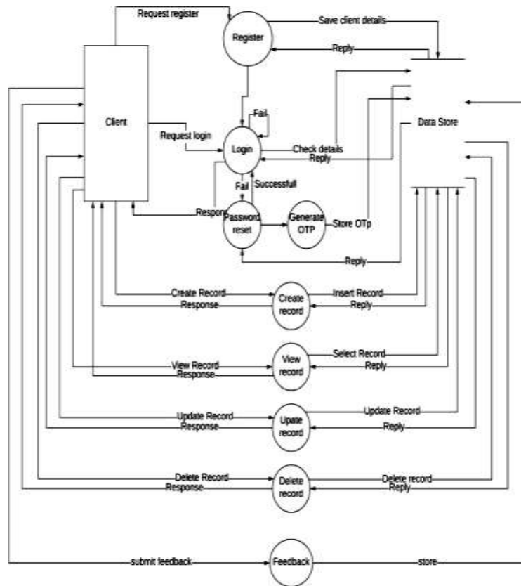
Fig. 1 DFD Level 2
